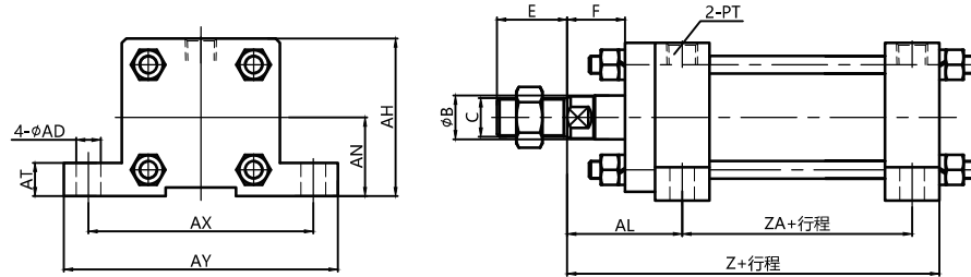
标准HOB+LB型 前后脚脚座型
