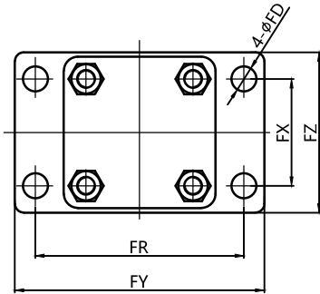
标准HOB+FA型 前法兰型
