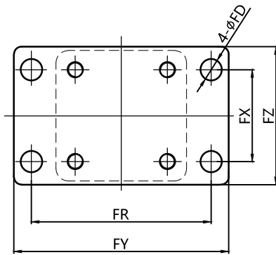
标准HOB+FA型 后法兰型
